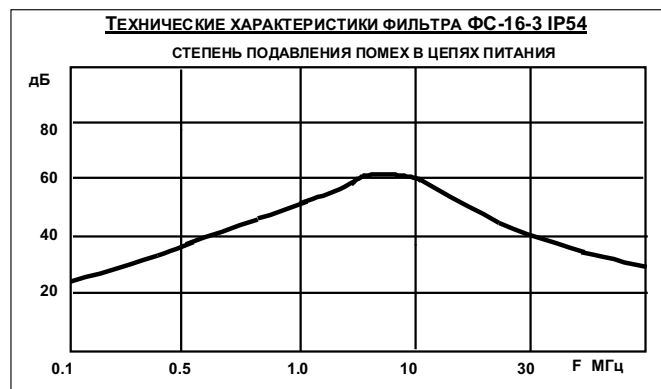
Рис.2. График АЧХ фильтра ФС-16-3 IP54 .
