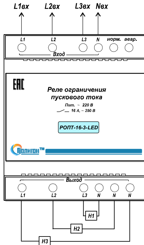
Рис.1. Типовая схема подключения РОПТ-16-3-LED.
